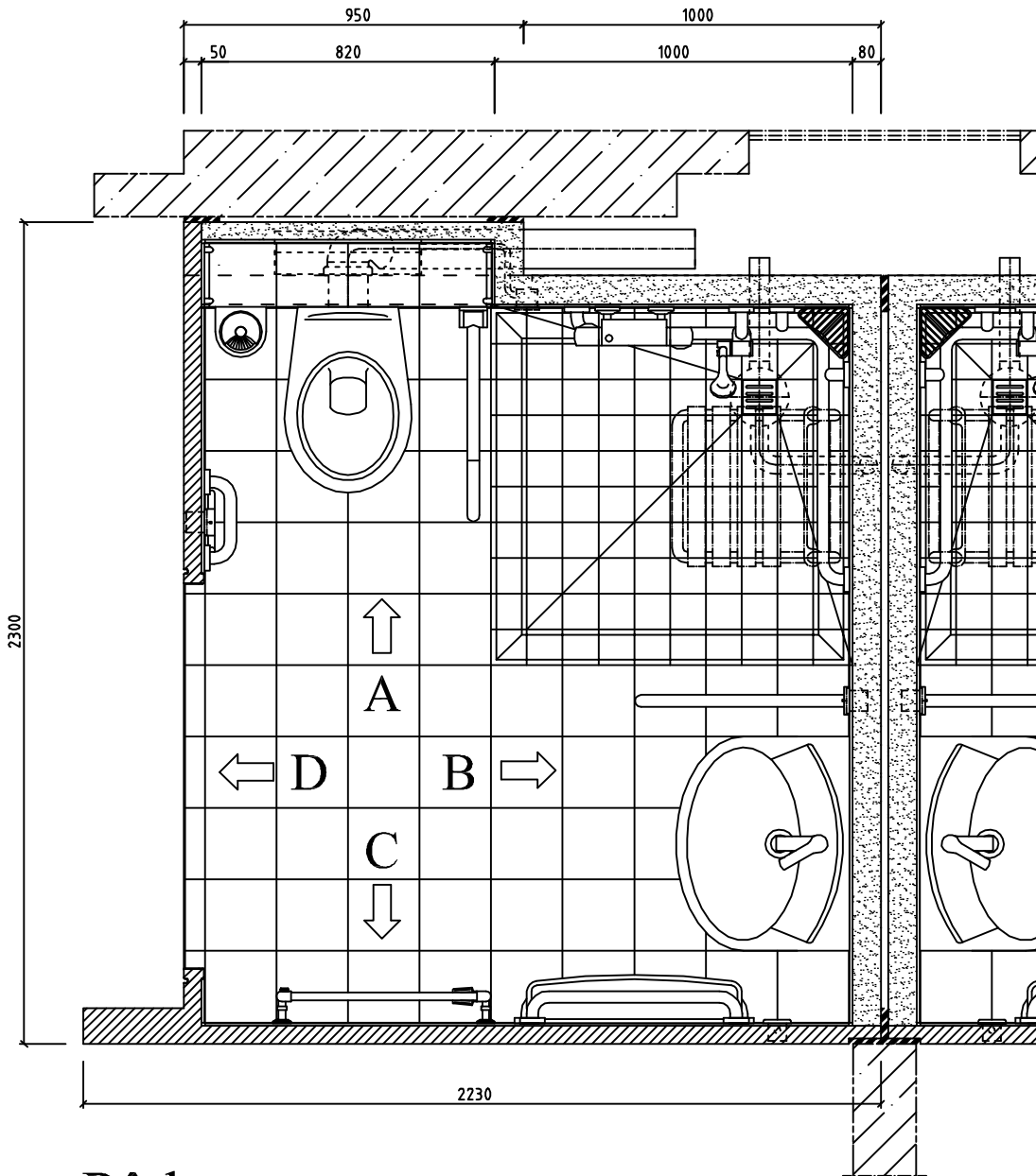
Pôdorys
